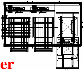
PCB Picker and Contactless Centering PCB 提取臂 和 非接触式定心机构
